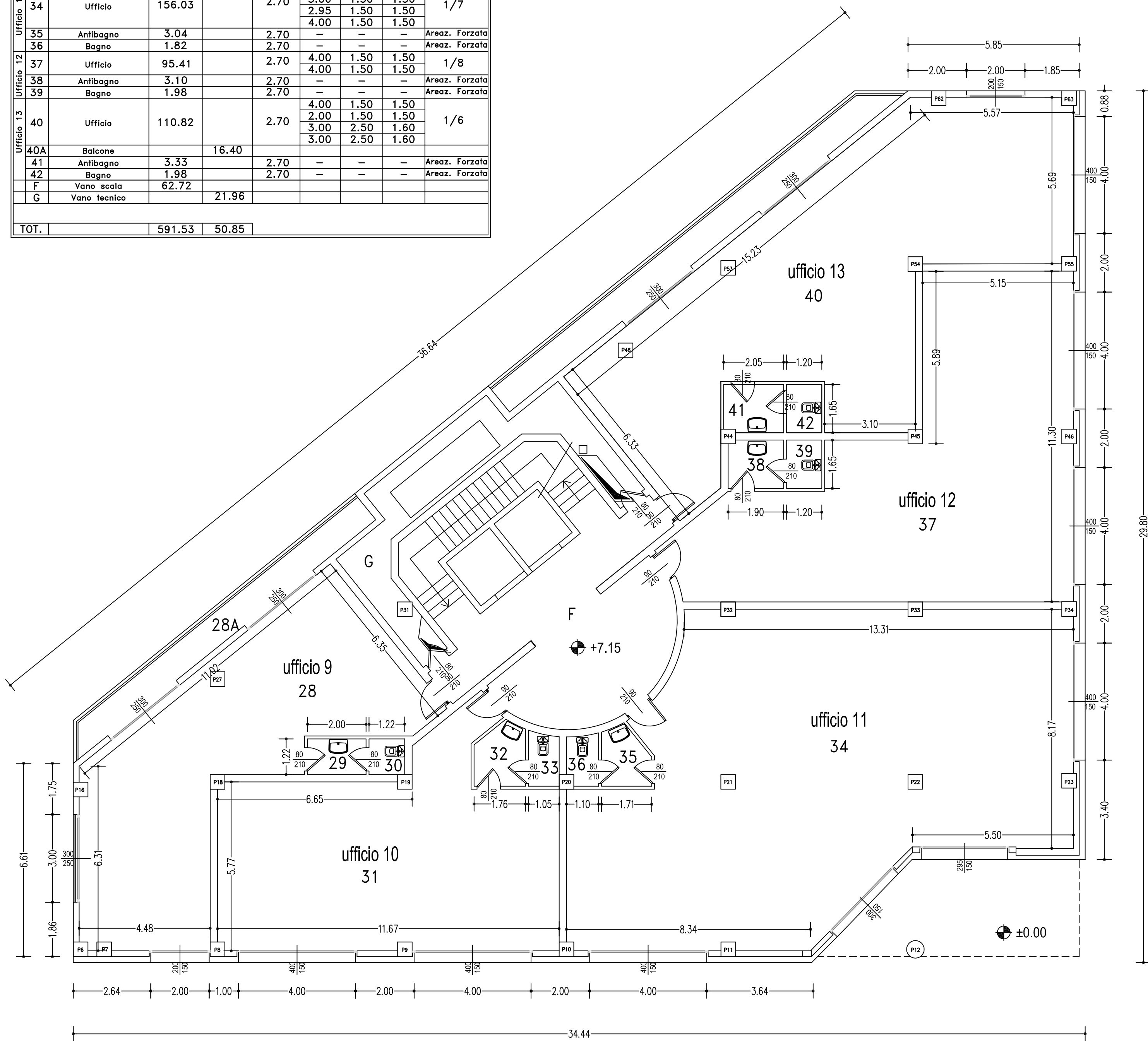
Planimetria piano secondo
