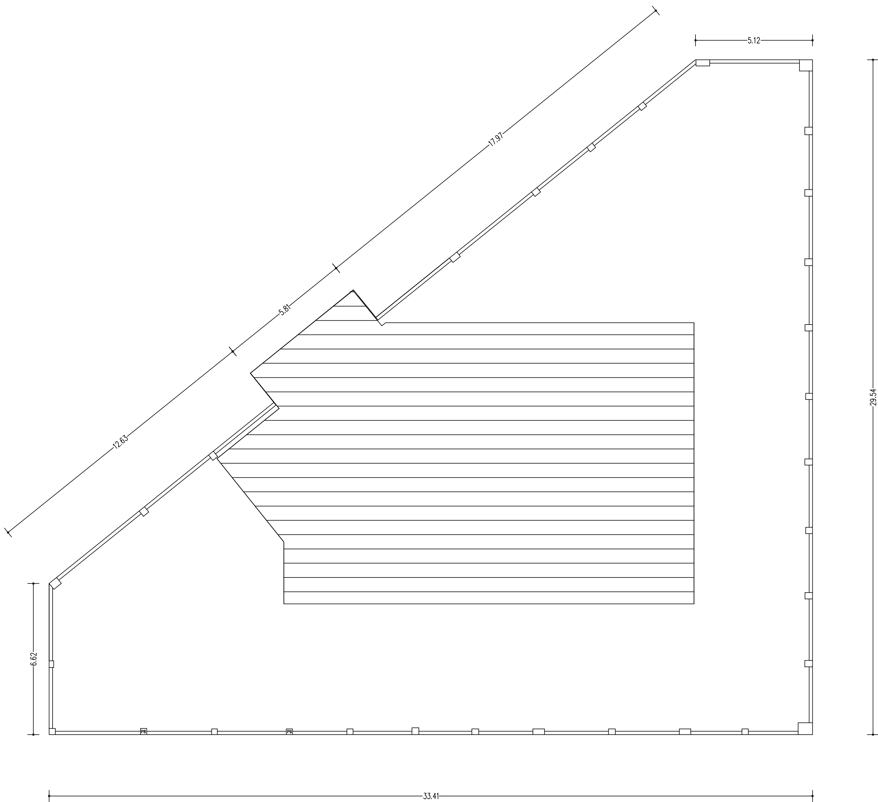
Planimetria piano copertura
