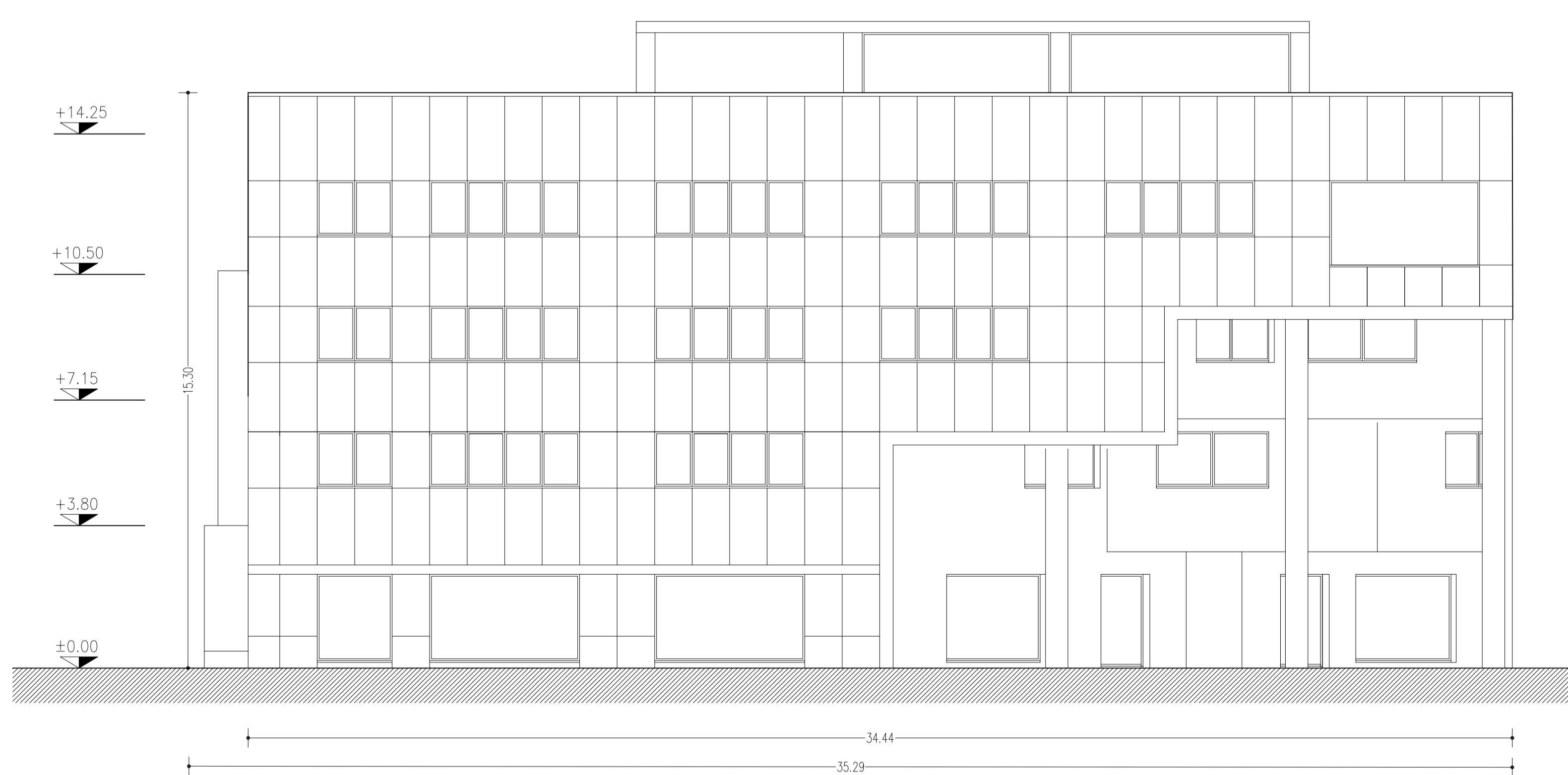
PROSPETTO EST
