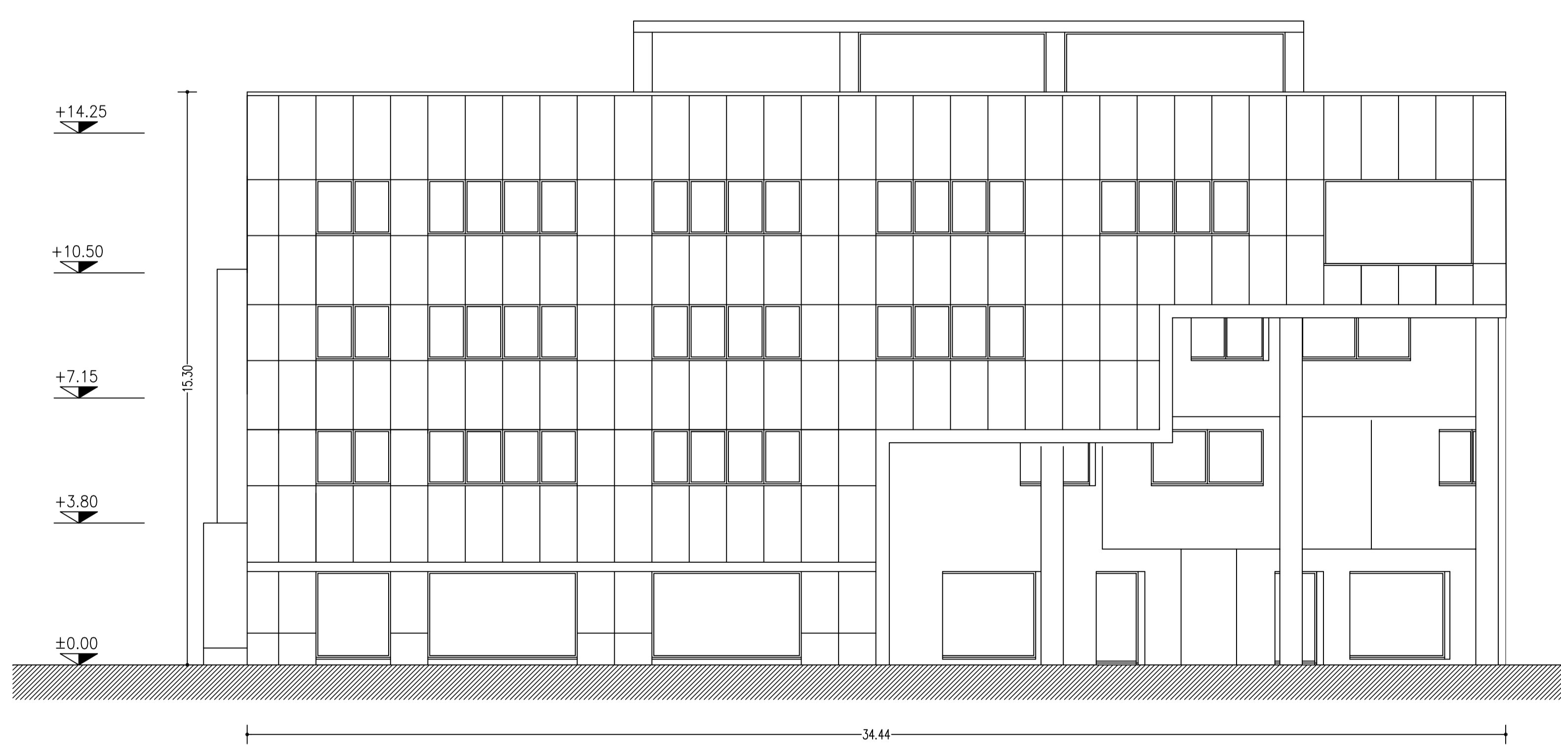
PROSPETTO EST
