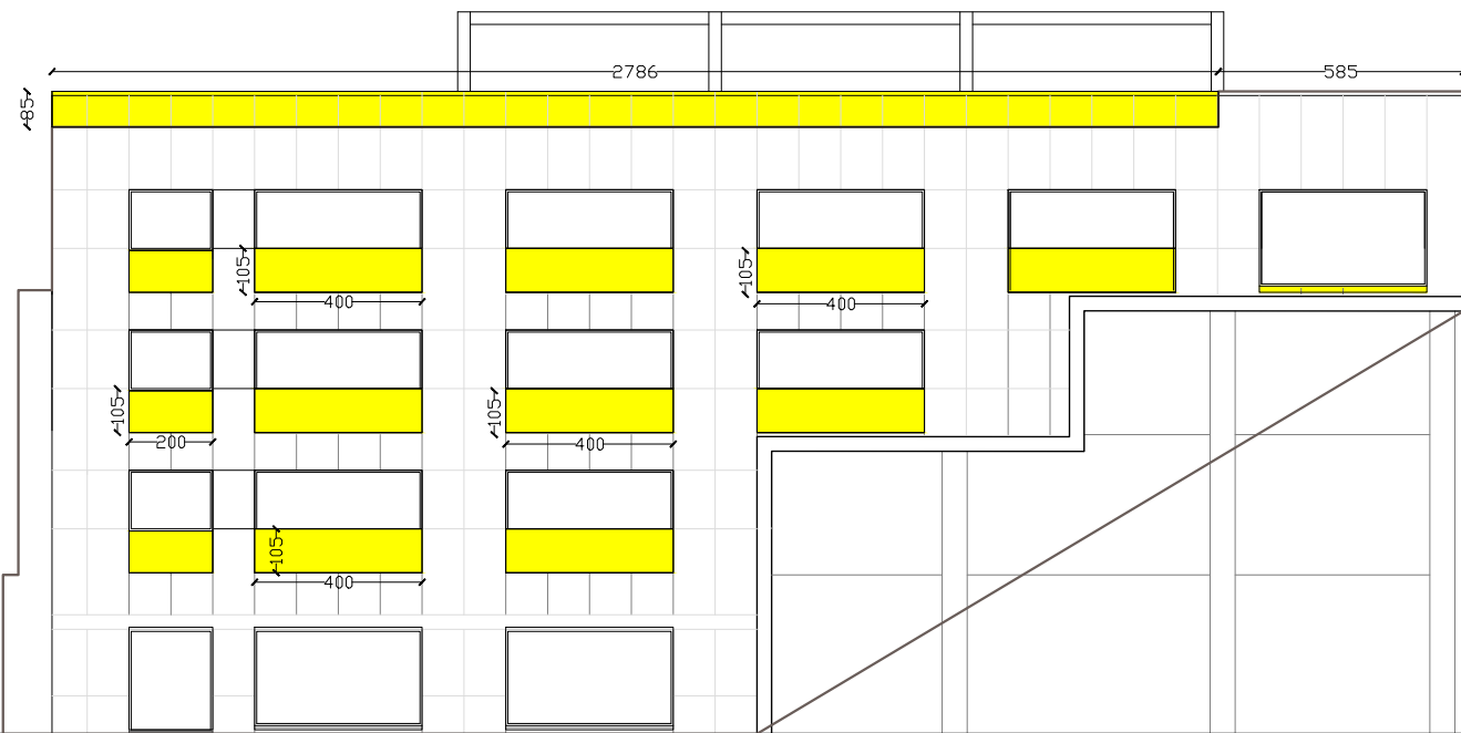
PROSPETTO EST DEMOLIZIONI
