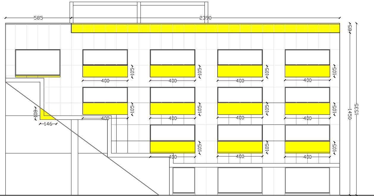
PROSPETTO NORD DEMOLIZIONI
