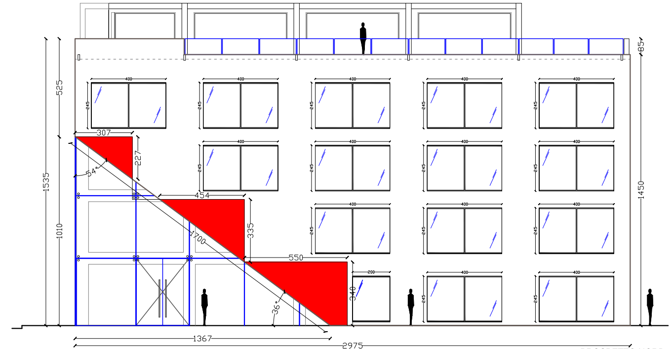
PROSPETTO NORD COSTRUZIONI
